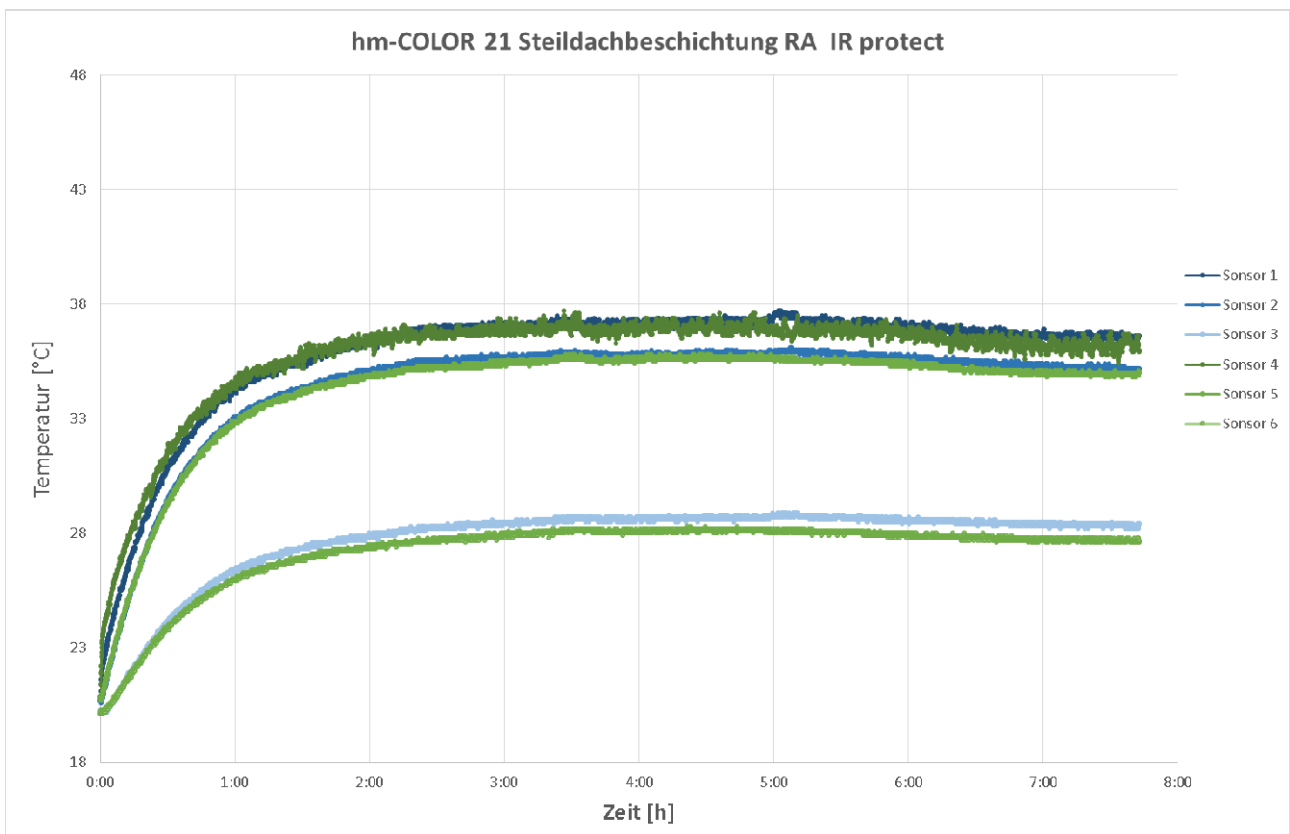
Abbildung 3: Temperaturverlauf von hm-COLOR 21 Steildachbeschichtung RA IR Protect
