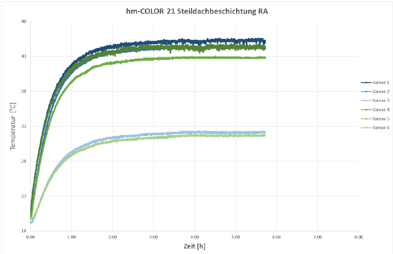
Abbildung 2: Temperaturverlauf von hm-COLOR 21 Steildachbeschichtung RA
